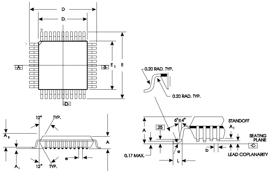
TQFP Package
